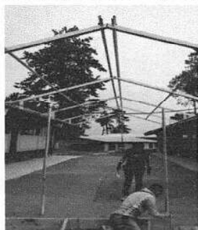
Foto 3: Suministro e instalación de costaneras de metal para entechado de pasillo de aulas.
